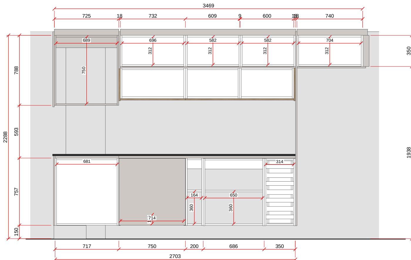
VISTA A - ESC. 1:25
